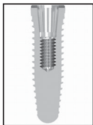
Roscas externas e internas de um implante.
